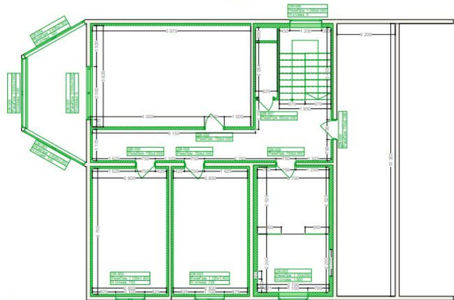
План монтажа 2 этаж
