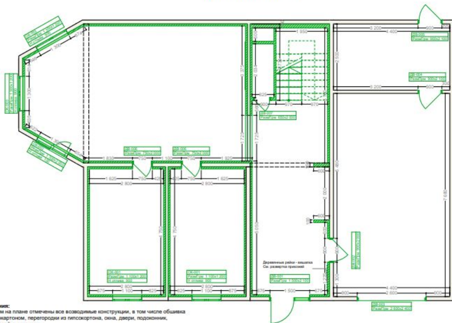
План монтажа 1 этаж
